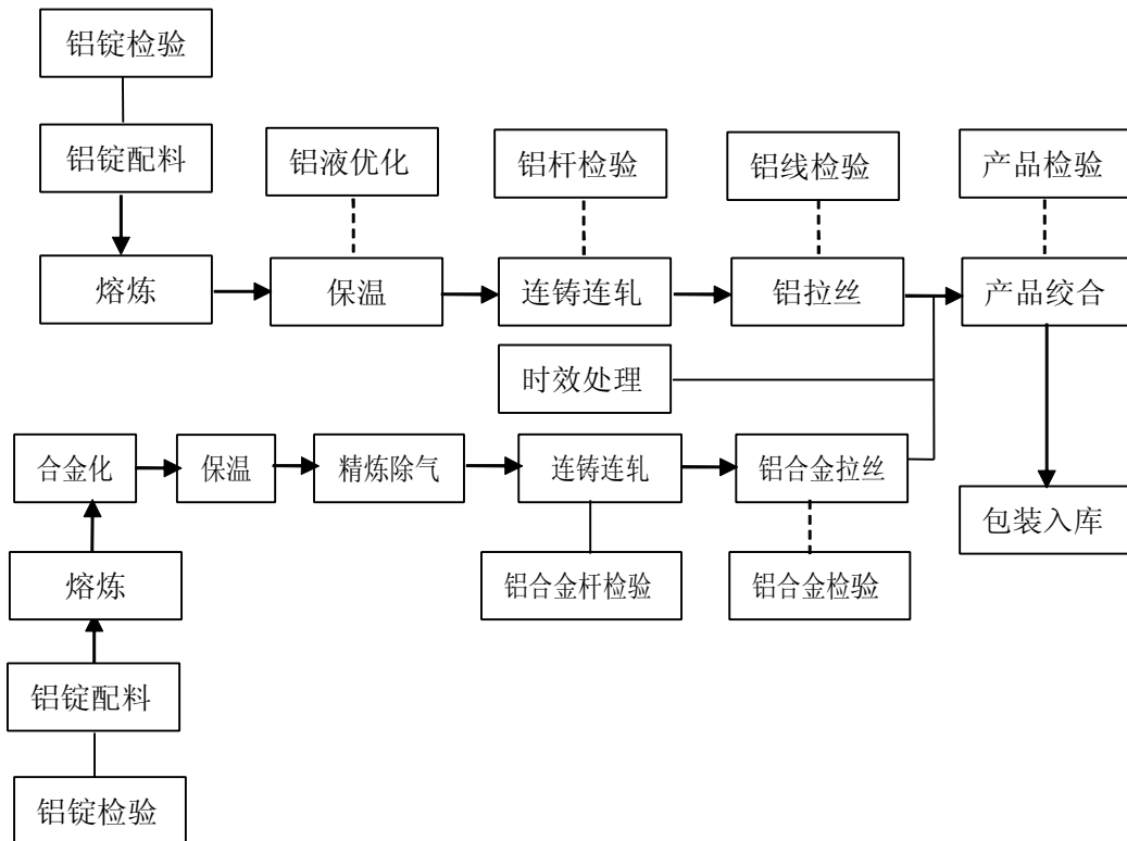
图 3 铝合金芯铝绞线主要工艺流程图
