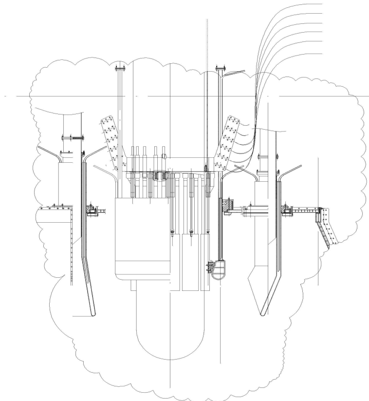
图2 新型导电铜瓦把持器结构示意图
