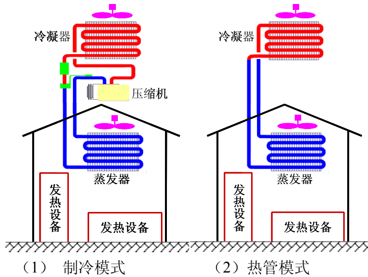
图 1 热管/蒸汽压缩复合制冷技术示意图
